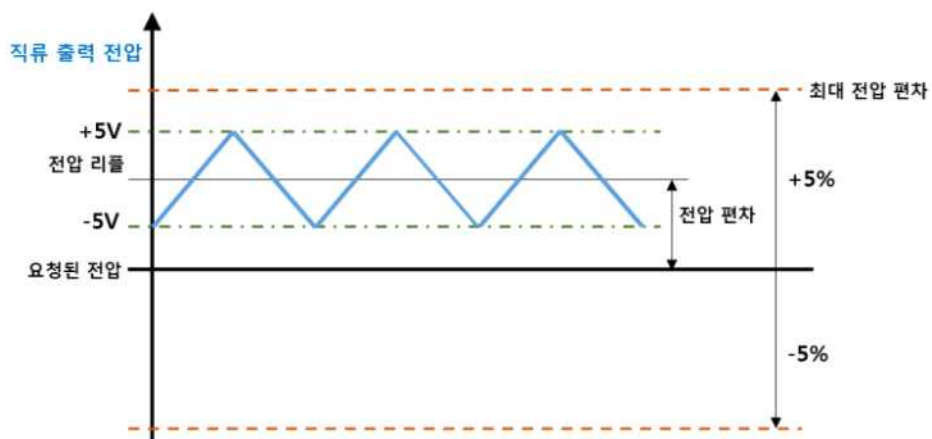
[그림 2] CVC 최대전압 편차 및 리플
