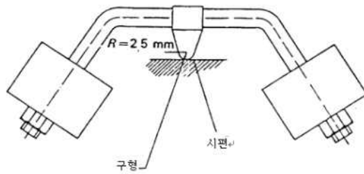
[그림 1] 구슬 압력 장치
