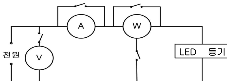
[그림 1] 입력 전류 및 입력 전력 측정 회로
