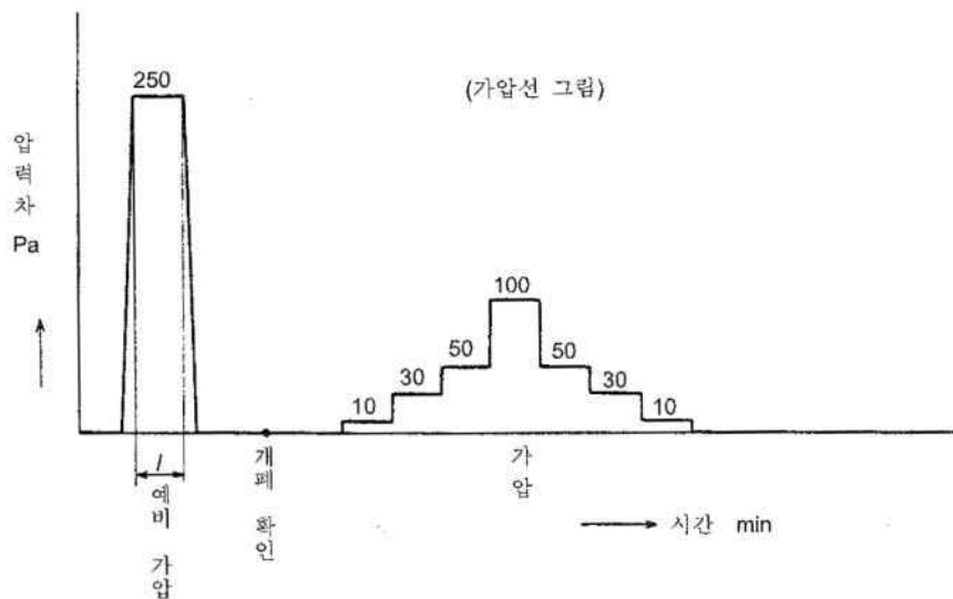
[그림 7] 기밀성 시험 순서
